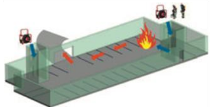
1 Ein- Ausfahrt vorhanden, Angriff über den Treppenraum, Belüften über den Gebäudeeingang mittels MGV, Abluftöffnung ist die Ein-Ausfahrt (Foto: Die Freiwillige Feuerwehr 4/2013)
