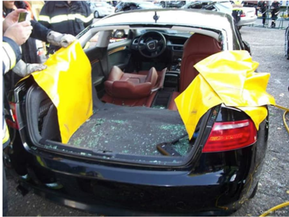
Hecköffnung (Kofferraum)
