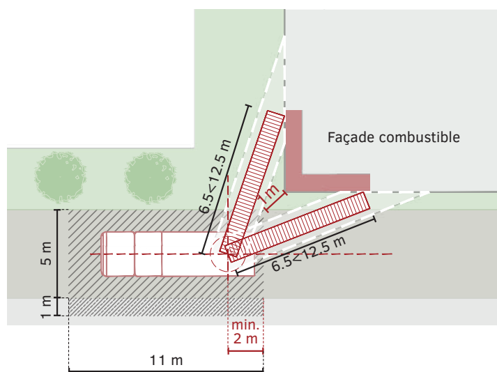
Schéma de principe - Surface d'appui avec façade combustible en angle
