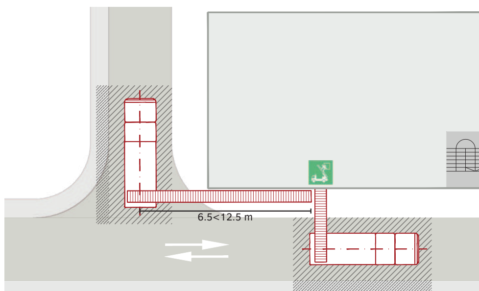
Schéma - Voie d'évacuation accessoire sur bâtiment moyen
