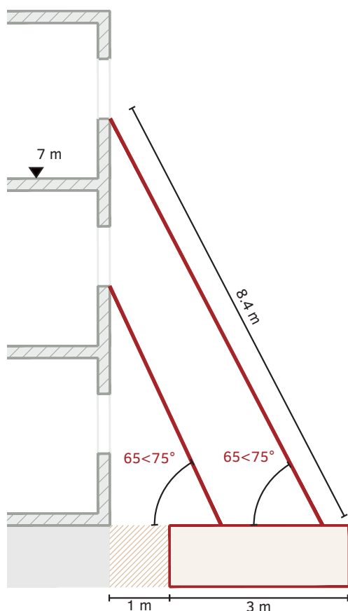
Schéma - Surface d'appui ponctuelle pour échelle portable
