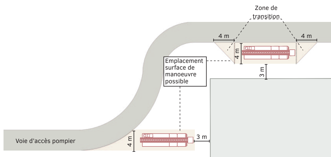
Schéma - Illustration des surfaces de manoeuvre
