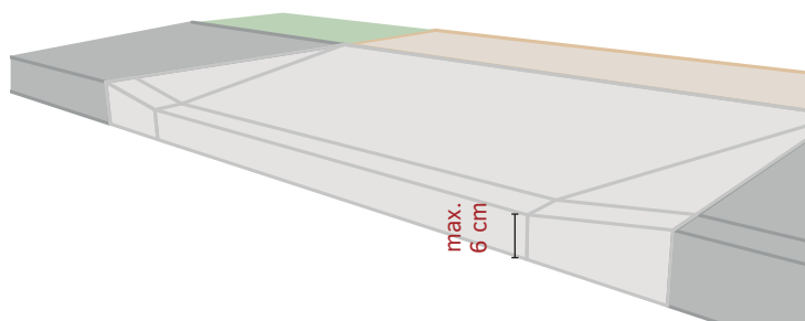
Schéma - Abaissement de trottoir pour voies d'accès pompiers
