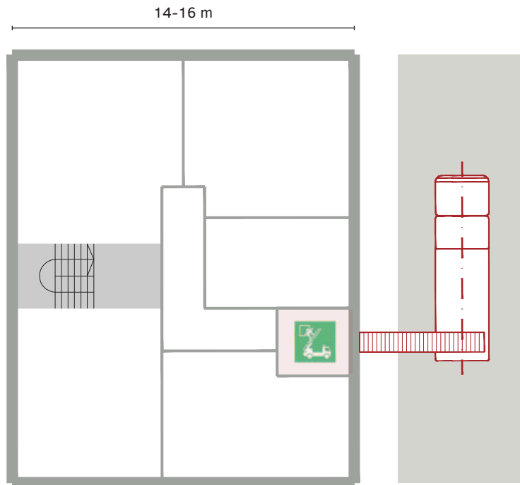
Schéma - Voie d'évacuation accessoire avec espace commun
