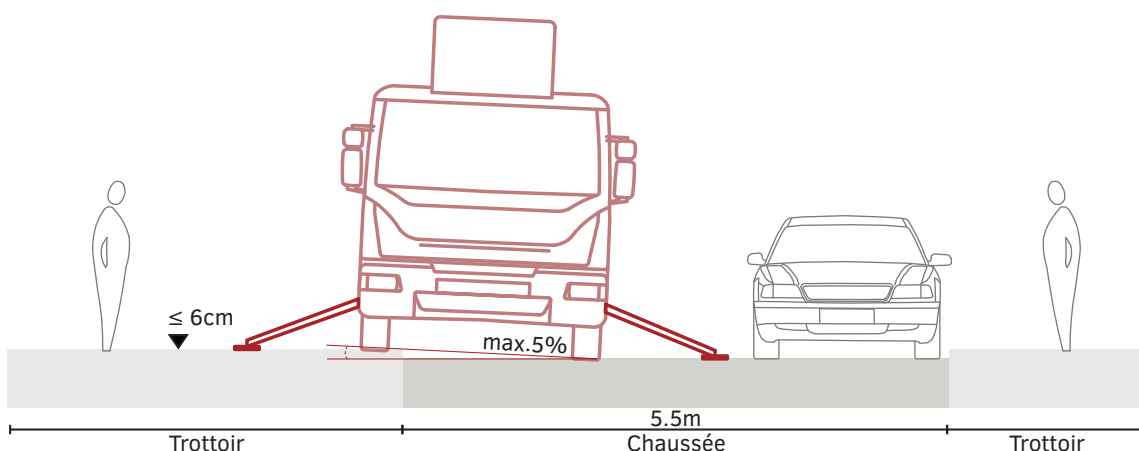
Exemple d'application - Surface d'appui sur trottoir inférieur ou égal à 6 cm
