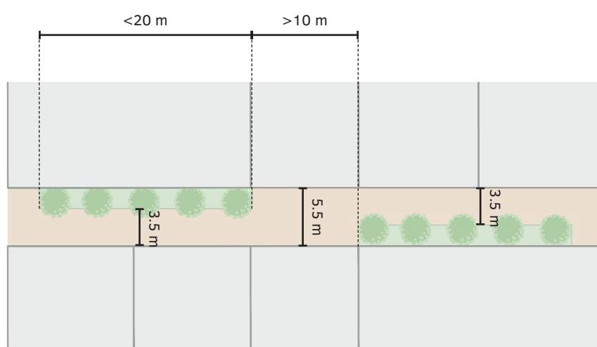
Schéma d'aménagement d'un apaisement de circulation
