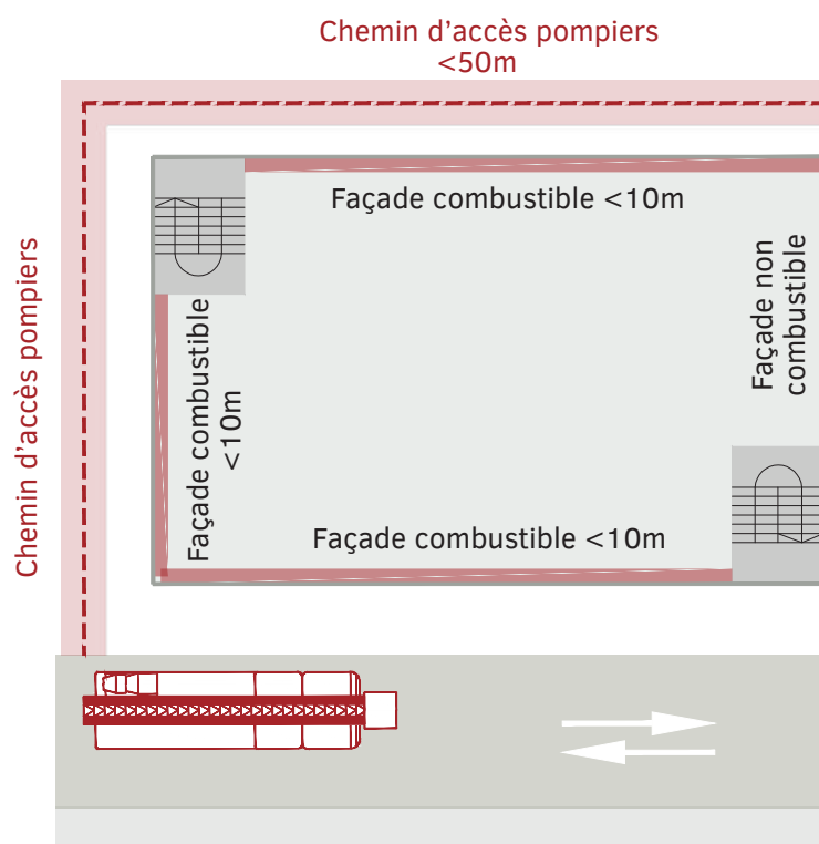
Schéma - Extinction de façades combustibles sur hauteur de façade jusqu'à 10 m
