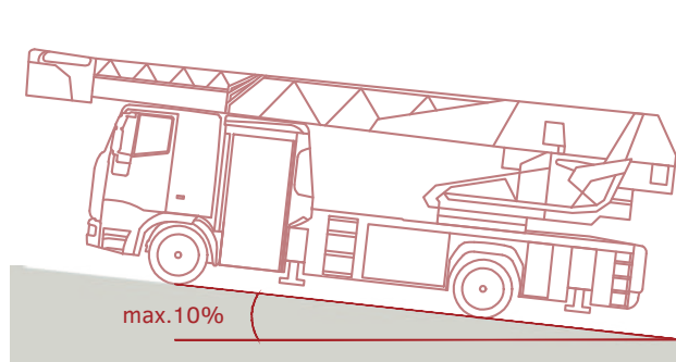
Schémas - Déclivités surface de manœuvre et d'appui
