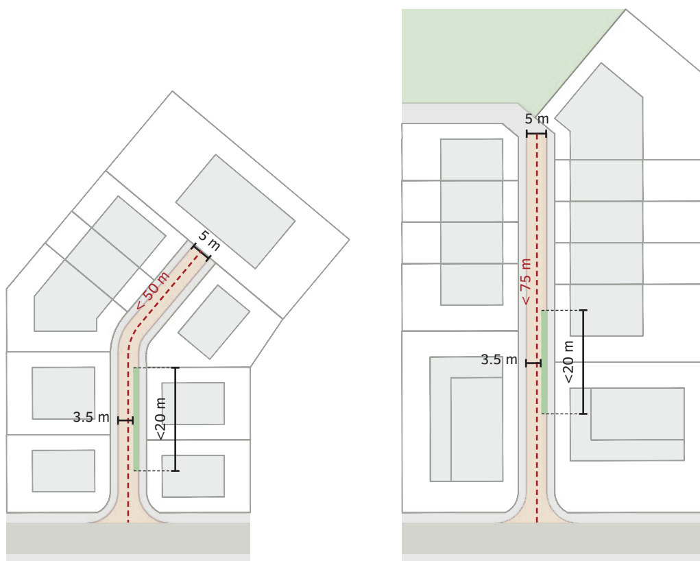
Schéma – Voie sans issue
