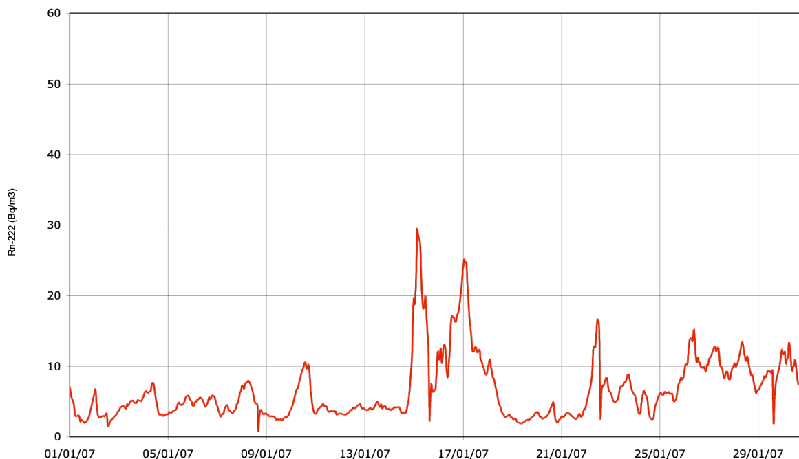
Concentration en radon dans l'air à Luxembourg-Villa
